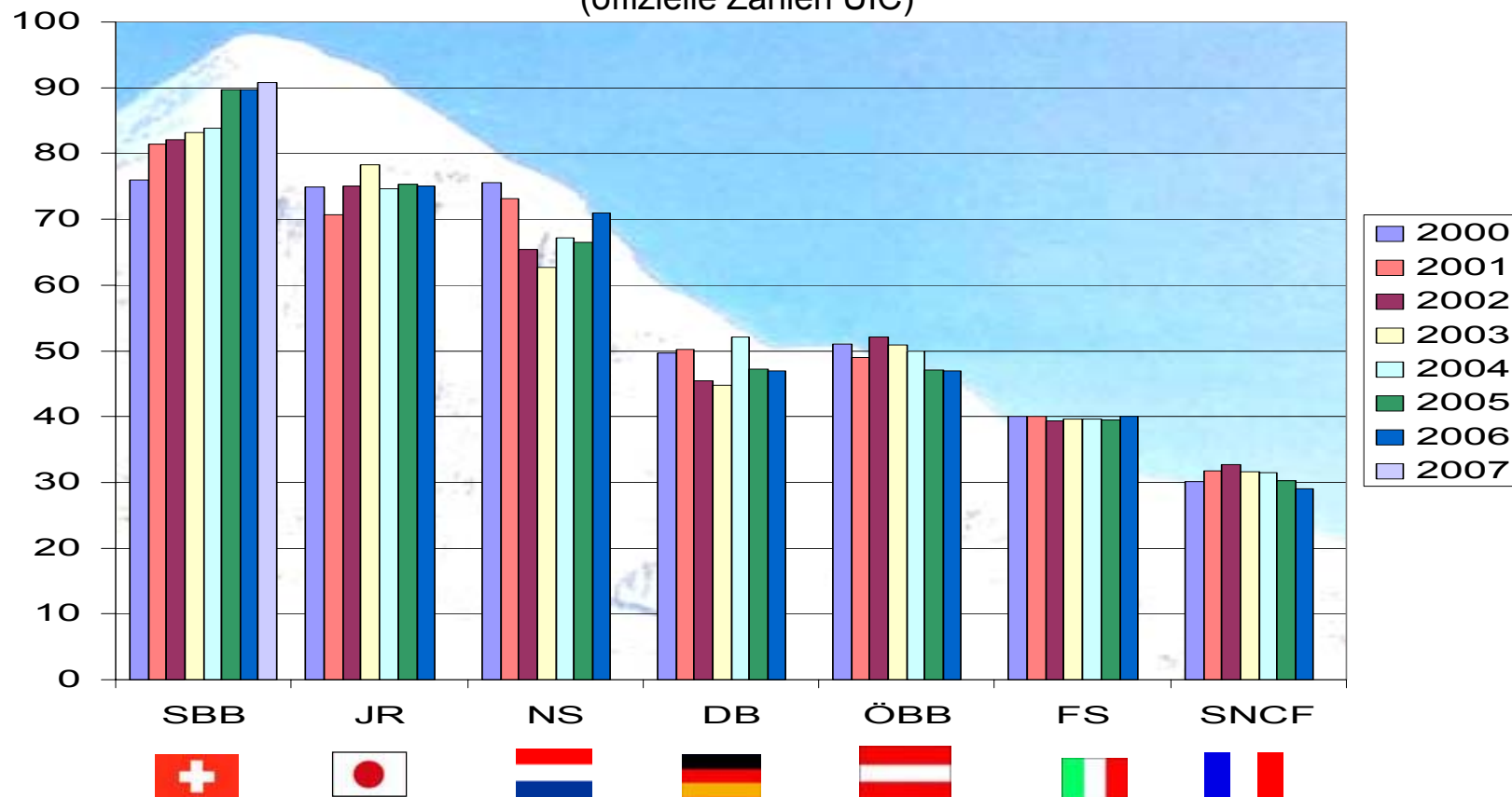
Netznutzungseffizienz: Zugkilometer pro Kilometer Schiene im Tag (offizielle Zahlen UIC)
